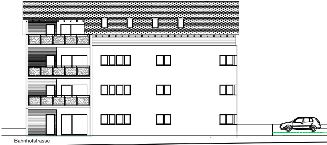
Süd-Ostfassade
