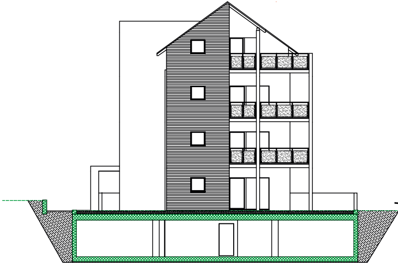
Süd-Westfassade
